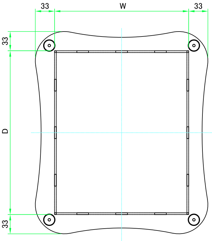
Wパネル1 / W panel 1
