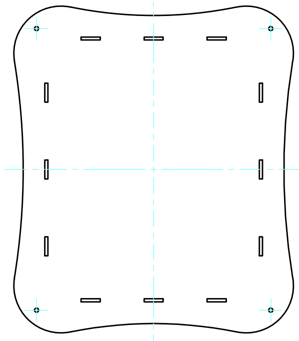
下カバー裏面 / Bottom cover Backside
